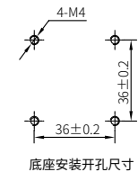
底座安装型LW39-16B M-□-□/□□□
