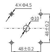
客户安装开孔尺寸
