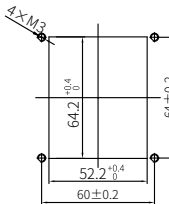
客户安装开孔尺寸
