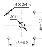
客户安装开孔尺寸
