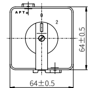
底座安装型LW39-25 M-□-□/□□□
