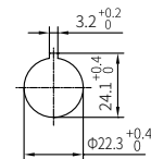
客户安装开孔尺寸
