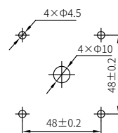
客户安装开孔尺寸
