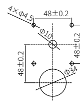
客户安装开孔尺寸
