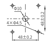
客户安装开孔尺寸
