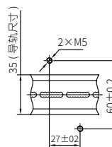
客户安装开孔尺寸
