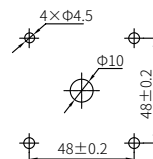
客户安装开孔尺寸
