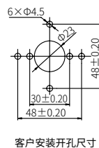
客户安装开孔尺寸
