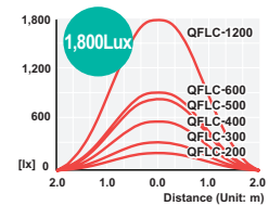
照度特征
