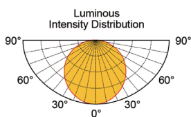
配光曲线图
