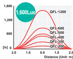
照度特征
